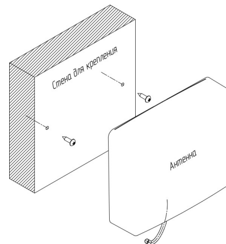
Схема 2 – Монтаж внутренней антенны
