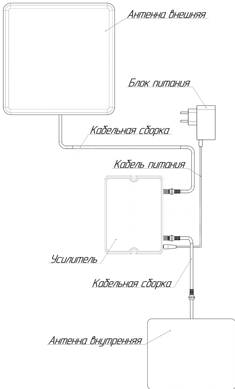
Схема 3 – Подключение комплекта
