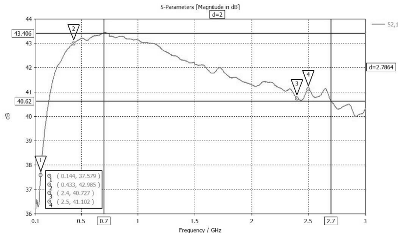
График 2 – Типовая амплитудно-частотная характеристика усилителя мощности
