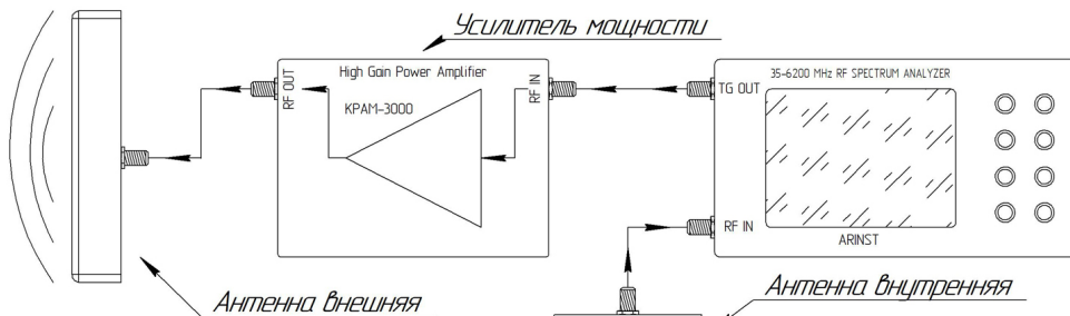
Схема 2 – Подключение усилителя
