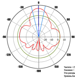
2700 МГц в вертикальной плоскости
