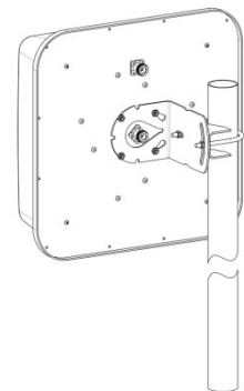
Монтаж антенны на мачте
