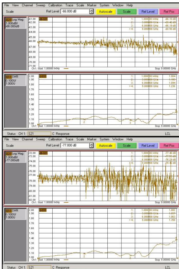
Графики для АЧХ - Log Mag, при отсчётом уровне равном -66 дБ, и для КСВ - SWR
